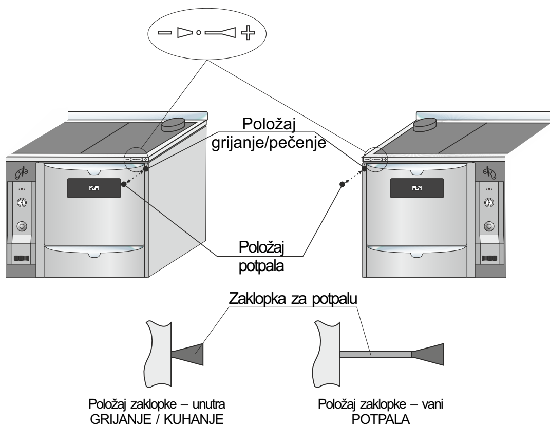
Slika 3. Uporaba zaklopke za potpalu kotla BIO-PEK B
