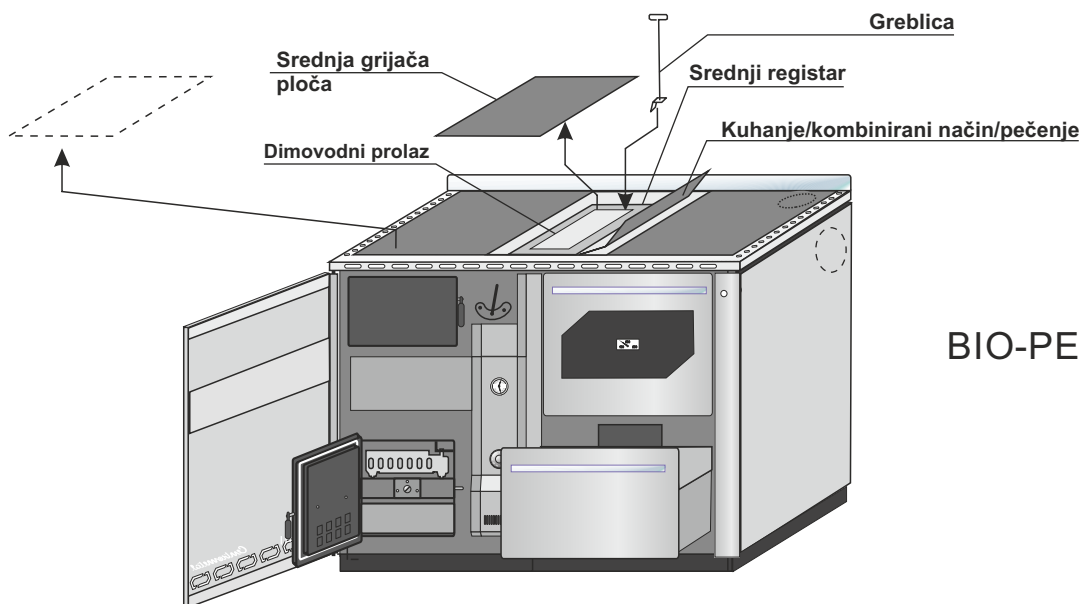
Slika 8. Čišćenje površina – kotao BIO-PEK B–D (vrijedi i za kotao BIO-PEK B–L)
