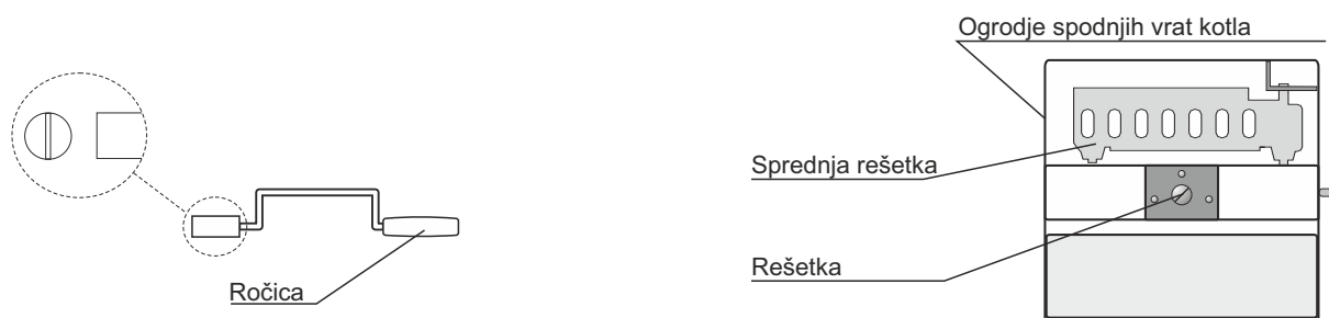
Slika 11. Sprednja rešetka in orodje za dvigovanje rešetke
