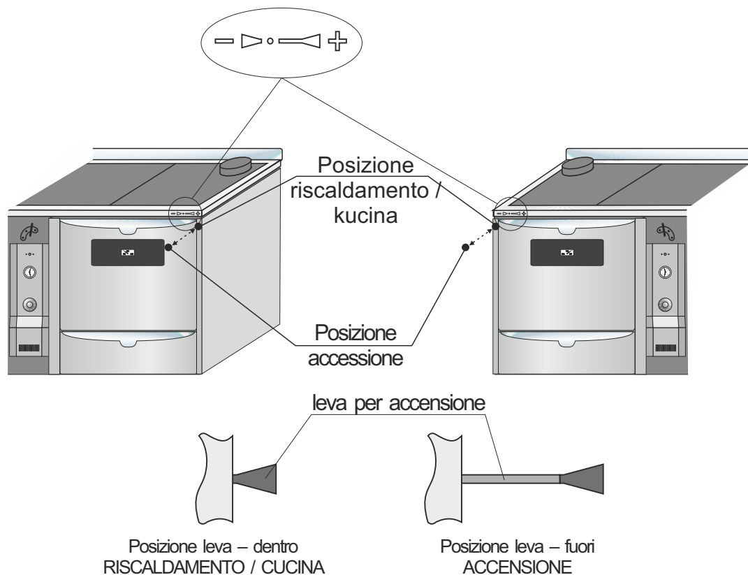
Foto 3. Uso per l'accensione della caldaia BIO-PEK B
