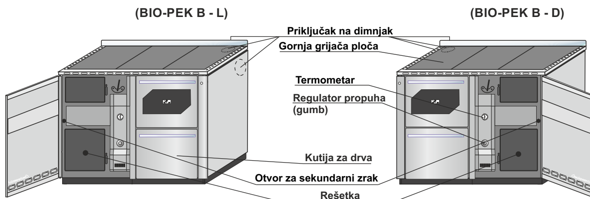
Slika 9. Osnovni dijelovi
