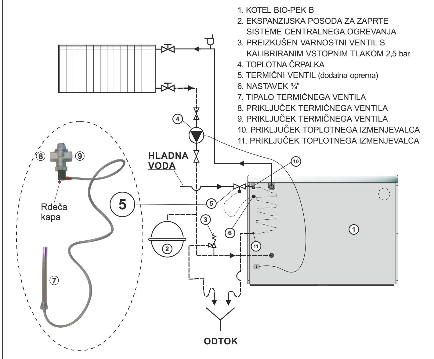
Diagram 2. Priklučki kotla BIO-PEK B–L (velja tudi za kotel BIO-PEK B–D)
