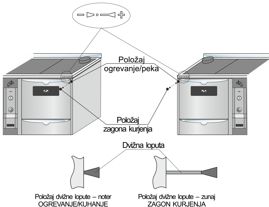
Slika 3. Uporaba dvizne lopute kotla BIO-PEK B
