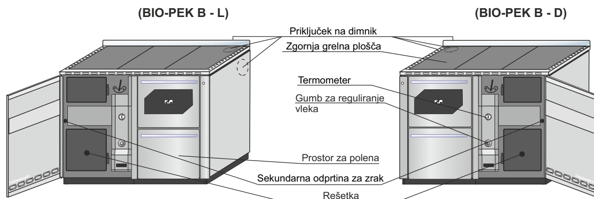
Slika 9. Osnovni deli
