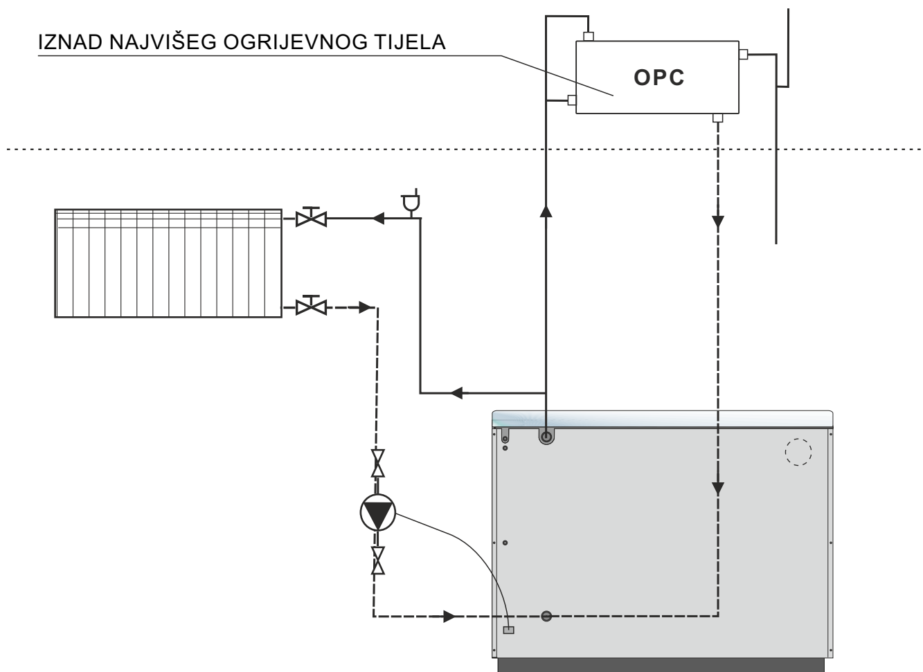
Shema 1: Spajanje kotla BIO-PEK B–L (vrijedi i za kotao BIO-PEK B–D)
